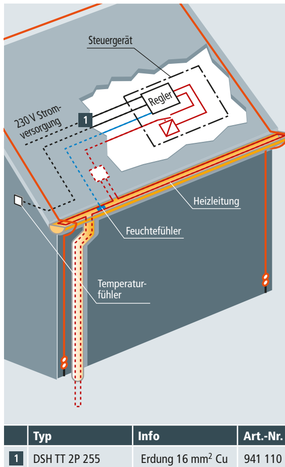
Bild 3 Blitzstromschutzbeschaltung bei eintrittsnaher Lage des Steuergerätes (Verlust wird akzeptiert) in einer baulichen Anlage mit äußerem Blitzschutz
