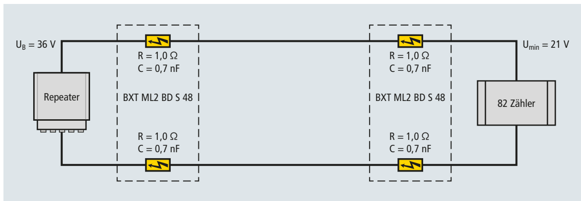
Bild 2 Leitungslängenreduzierung durch SPDs
