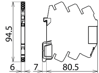
Maßbild DCO SD2 ME 24
