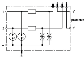
Prinzipialschaltbild DCO SD2 ME 12
