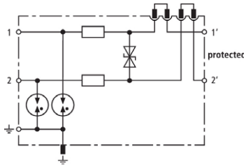
Prinzipialschaltbild DCO SD2 MD 48
