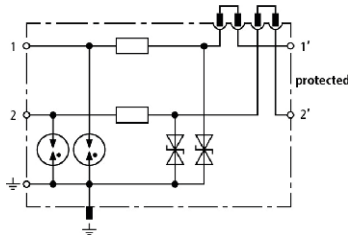
Prinzipialschaltbild DCO SD2 ME 24
