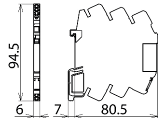
Maßbild DCO SD2 ME 12
