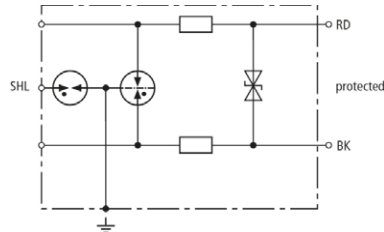
Prinzipialschaltbild DPI MD 24 M 2S
