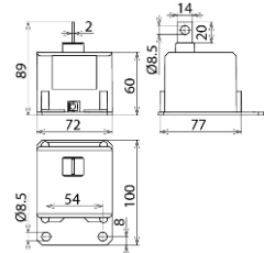
Maßbild DBM 1 255 S
