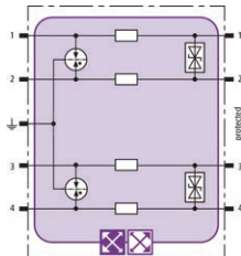
Principalschaltbild BXT ML4 BD HF 5
