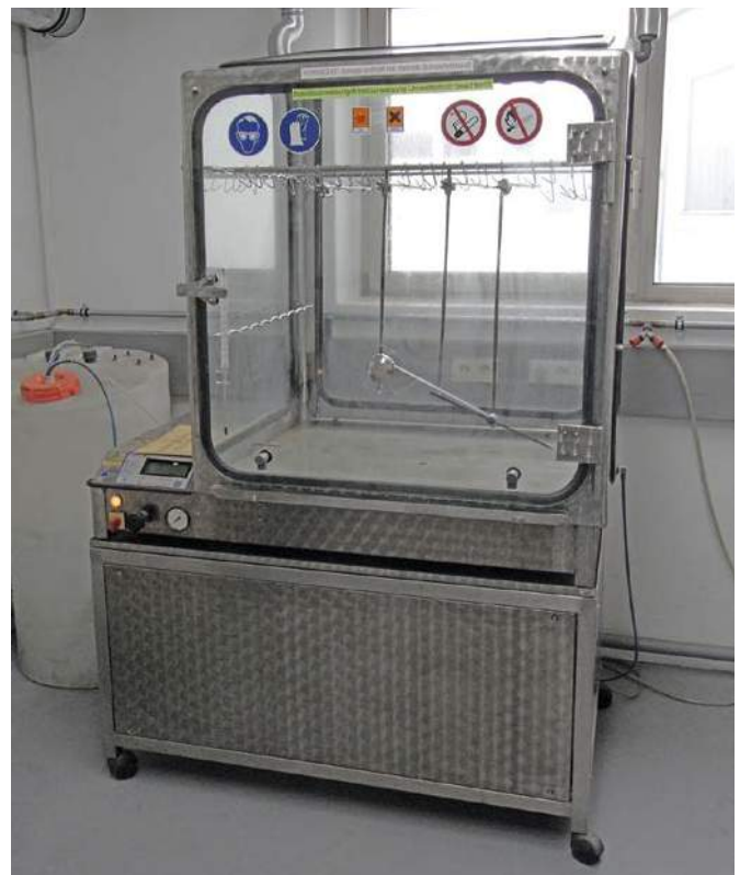
Bild 2: Prüfungen mit dem Kesternichgerät.
