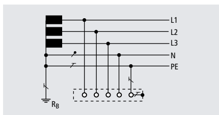
TN-S-System 230 / 400 V
