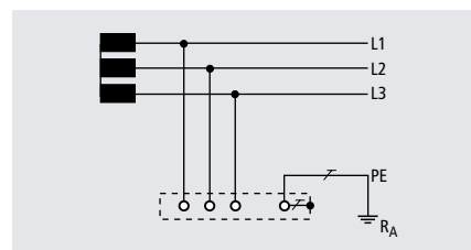
IT-System 230 V
