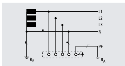
TT-System 230 / 400 V
