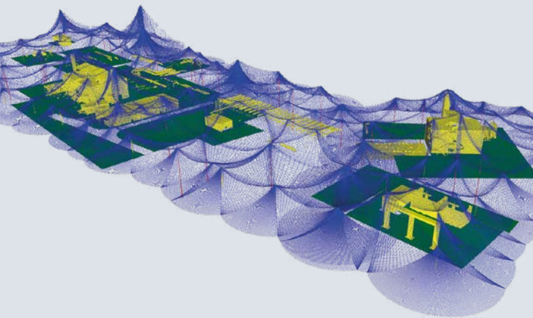
2 3D Blitzschutzkonzept – Schutzraumdarstellung einer Verdichterstation
