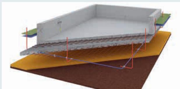
基础接地极
