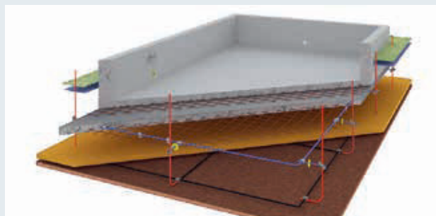
环形接地极
